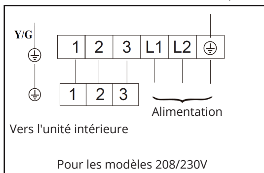
Schéma de branchement (208/230 V)
