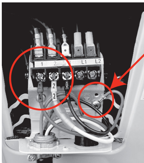
Branchement du fil de terre
